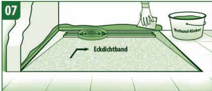
Eckdichtband im Eckbereich verlegen. (Alternativ Vlies-Randüberstand)
