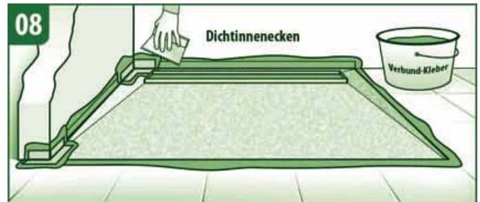
Im Eckbereich sind zwingend Dichtinnenecken zu verwenden, da dort das Dichtband eingeschnitten werden muss.
