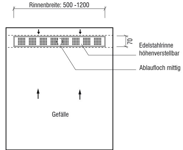
Draufsicht Duschelement: (Maße in mm, Maßstab 1:15)
